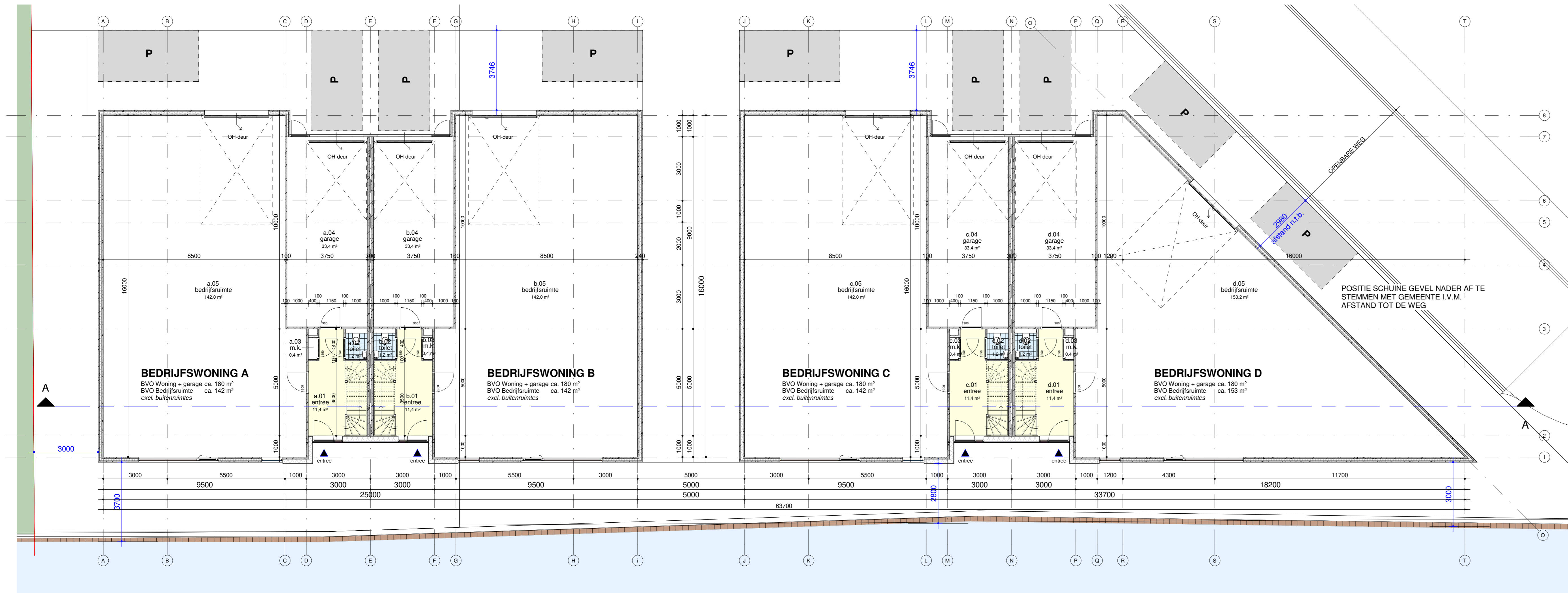
begane grond 1:100
