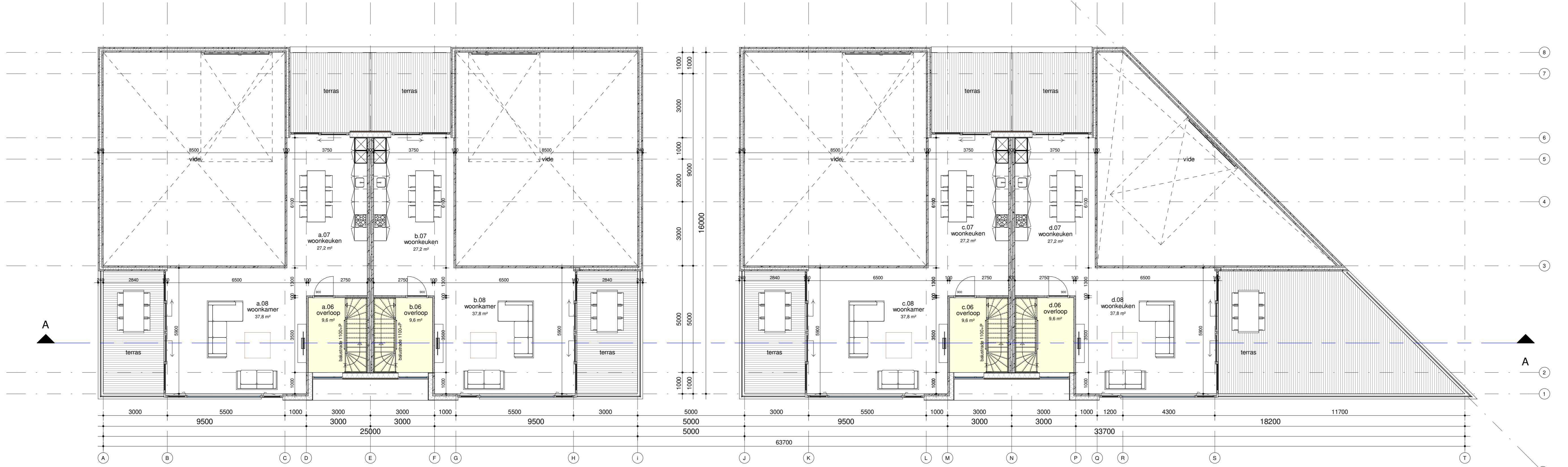
eerste verdieping 1:100
